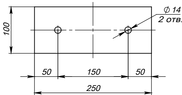
Поз.1 (Пластина)
