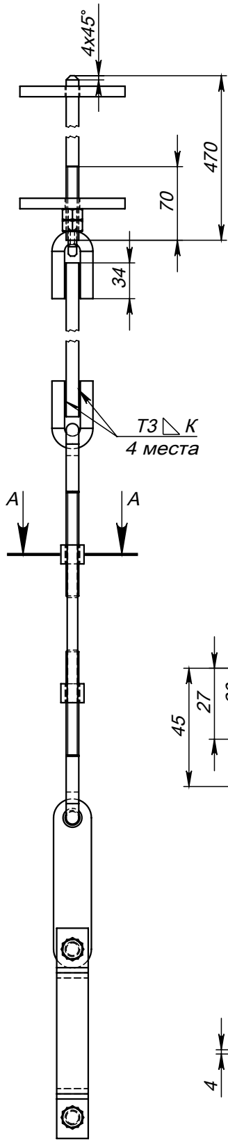
Поз.12 (Полухомут)
