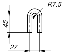
Поз.4 (Ушко)
