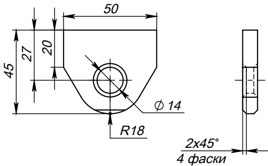
Поз.3 (Проушина) 1:2
