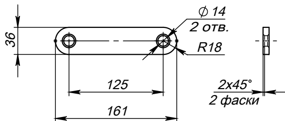
Поз.11 (Серьга)
